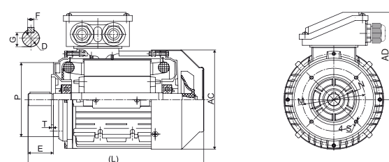
Figure 4 IM B14
