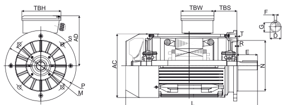
Figure 3 IM B5
