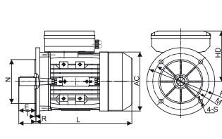
Figure 2 IM B5
