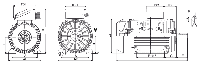
Figure 1 IM B3
