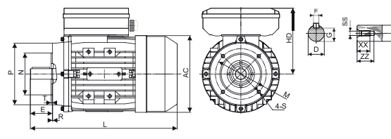
Figure 3 IM B14
