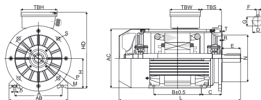
Figure 2 IM B35
