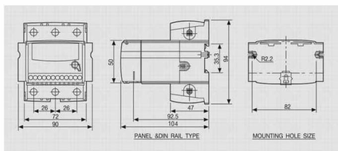
EOCR-PMZ
