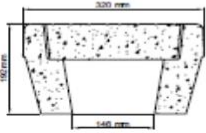
Hồ tiếp địa bê tông
