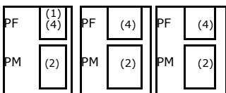
Liên động giữa 03 ACB di động (Withdrawable)
