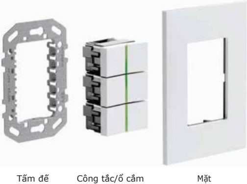
Cấu hình công tắc/ổ cắm dạng chữ nhật
