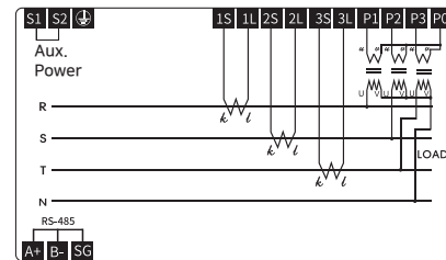
3 \phi 4W
