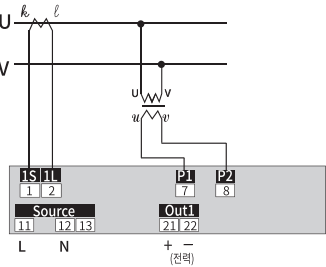
1P2W(LLType)
