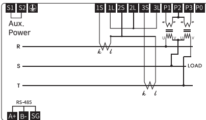
3 \phi 3W
