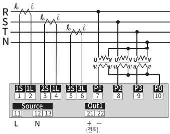
3P4W(LLType)
