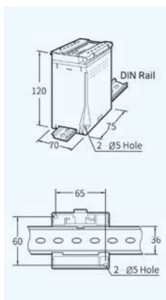
L Type(Unit : mm)
