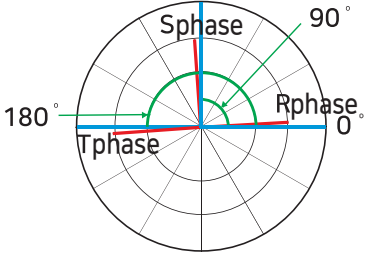
Example) Basic setting S-phase : 90 ° T-phase : 180 °
