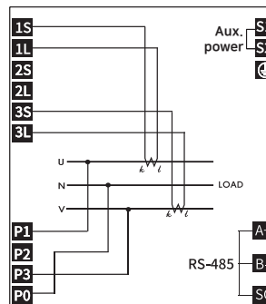
1P3W
